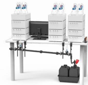
SymLine FLEX Gestão de Resíduos HPLC
